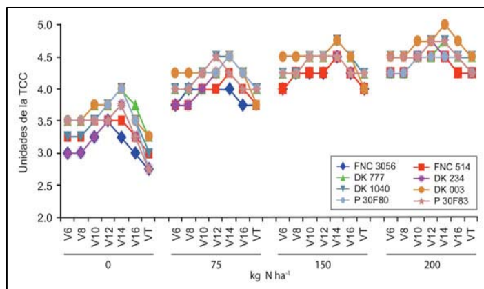
Figura 2. Efecto del material genético y de la dosis de N en la variación de unidades de lectura de la TCC en diferentes estados fisiológicos del maíz, Buga, Colombia, 2007.
