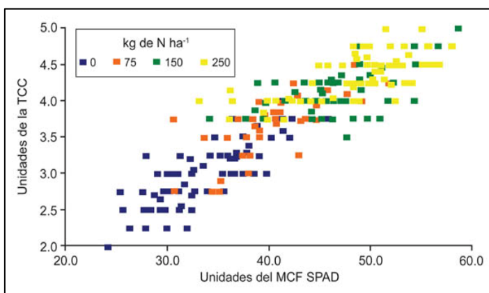
Figura 3. Correlación entre las unidades de lectura de la TCC y el MCF. Cada punto es el promedio de 10 lecturas.
