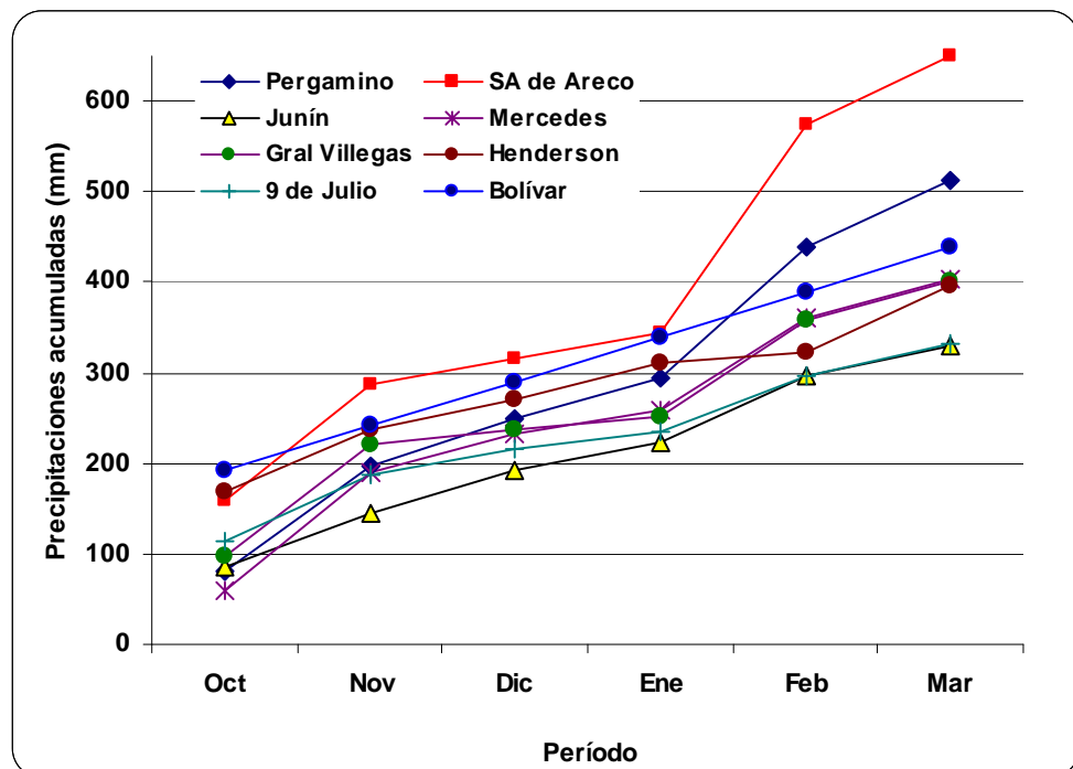
Figura 2: Precipitaciones acumuladas (mm) en períodos mensuales durante la estación de crecimiento de Soja.
